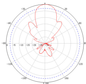
H-Plane
